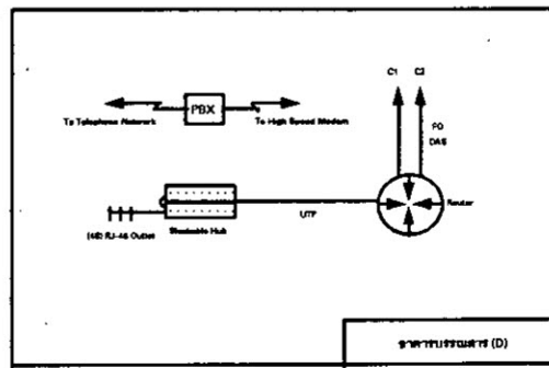
รูป 7.4D) แผนภาพแสดงการเชื่อมต่ออุปกรณ์เครือข่ายภายในอาคาร (D)
