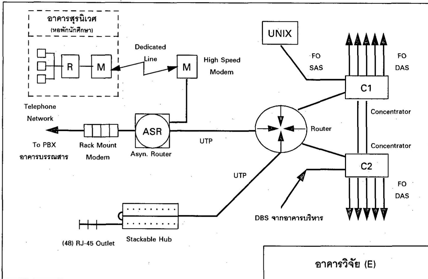
รูป 7.4(E) แผนภาพแสดงการต่อเชื่อมอุปกรณ์เครือข่ายภายในอาคารวิจัย (E)
