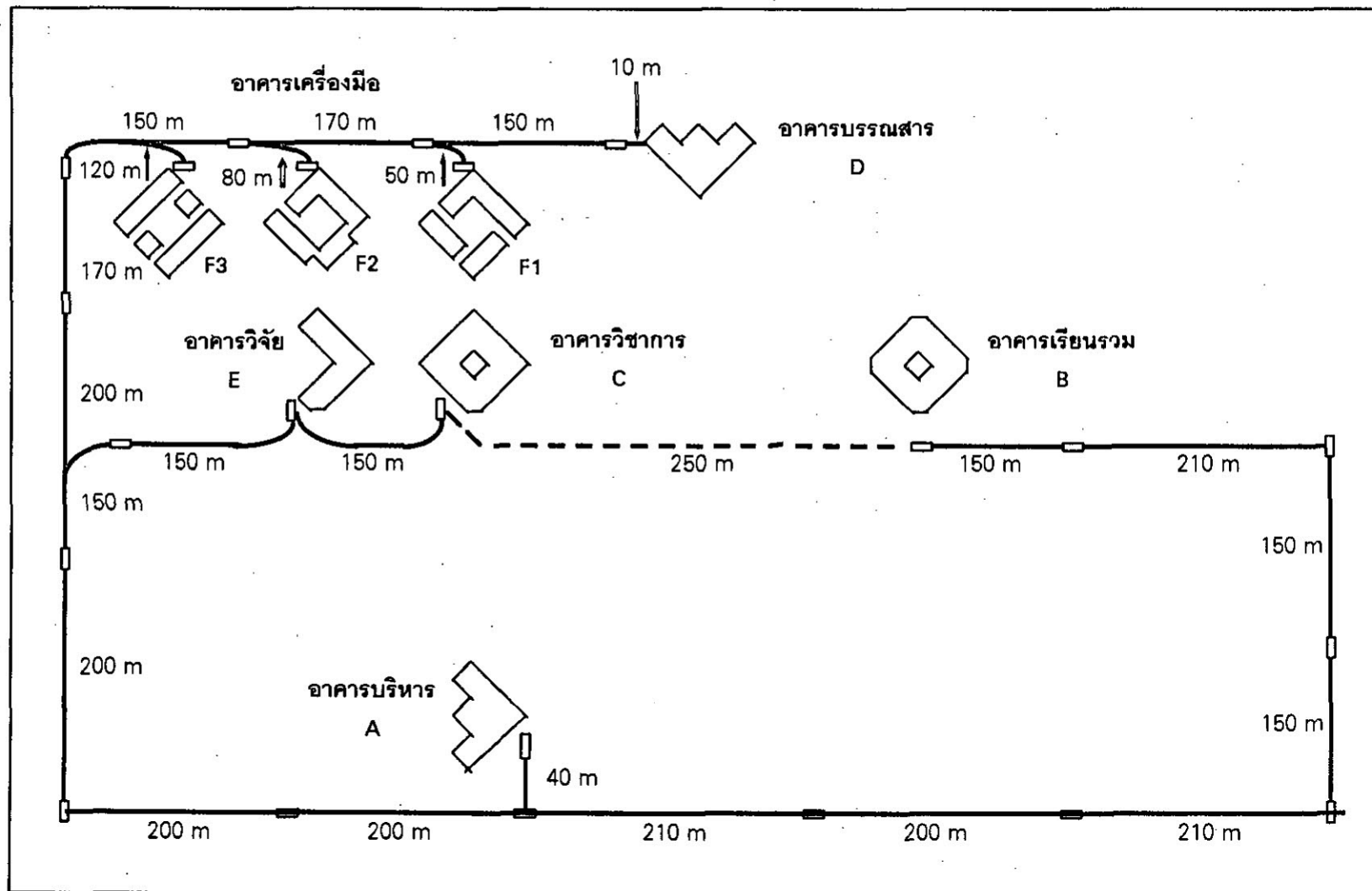
รูป 7.2 แผนผังอาคารและทางเดินที่ร้อยละสายโทรศัพท์มหาวิทยาลัย เส้นประแสดงแนวกำหนดในการติดตั้งที่ร้อยละสายเคเบิลใยแก้วนำแสง
