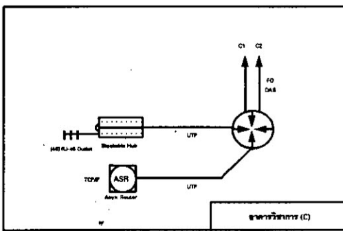
รูป 7.4C) แผนภาพแสดงการเชื่อมต่ออุปกรณ์เครือข่ายภายในอาคาร (C)
