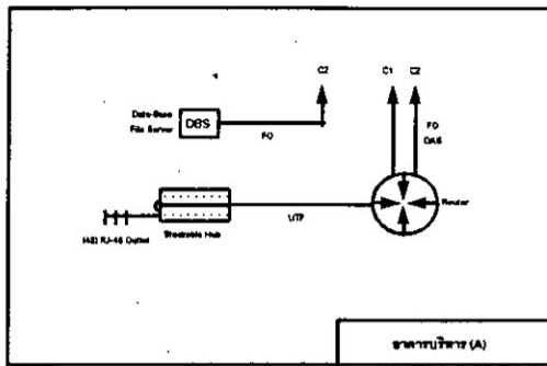
รูป 7.4A) แผนภาพแสดงการเชื่อมต่ออุปกรณ์เครือข่ายภายในอาคาร (A)
